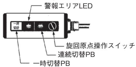
手元操作BOX SW配置図
