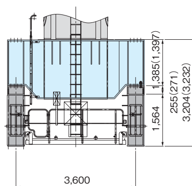
JCC-V720S形マスト取付状態
