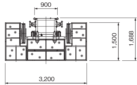
●連台平面図
