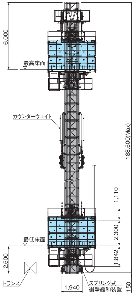
●主要寸法図
