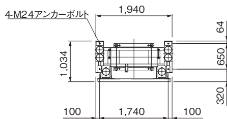
●ベース詳細図
