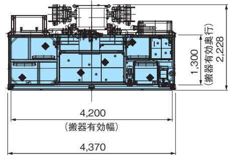
●搬器平面図
