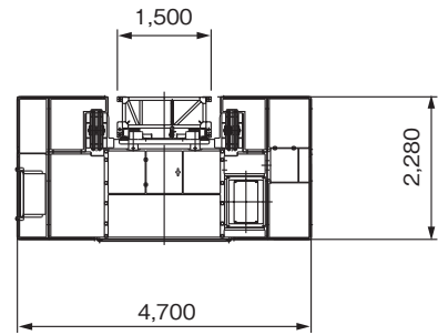
●連台平面図
