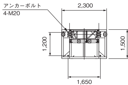
●ベース詳細図
