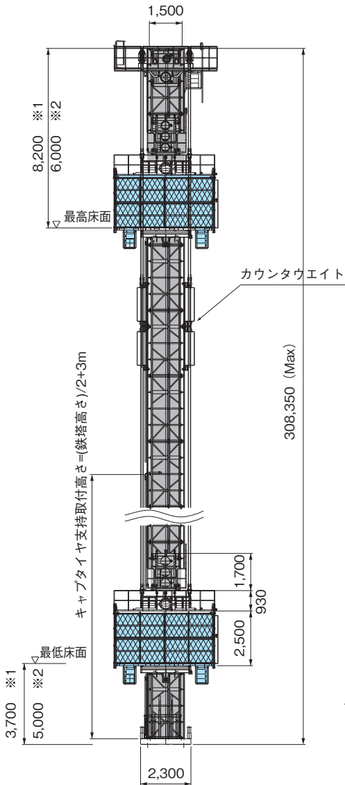
●主要寸法図
