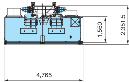
●搬器平面図
