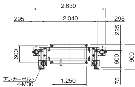
●ベース詳細図
