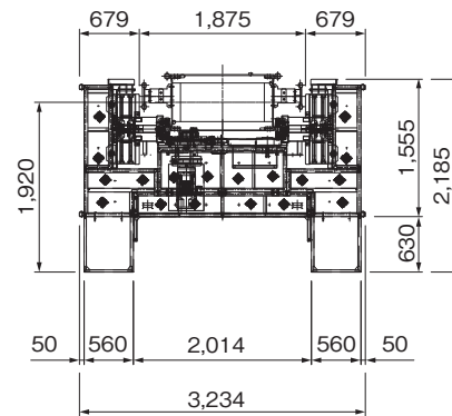
●搬器平面図
