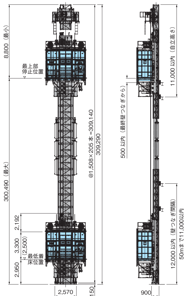
●主要寸法図
